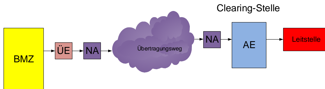
Abbildung 17: Getrennter Betrieb von Anschalteinrichtung und Übertragungseinrichtung
