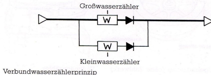
Verbundwasserzähler (Bild 16)
